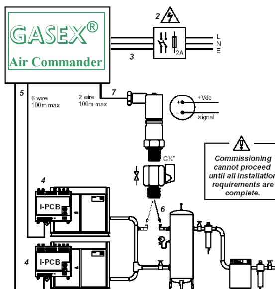
Typischer Aufbau
